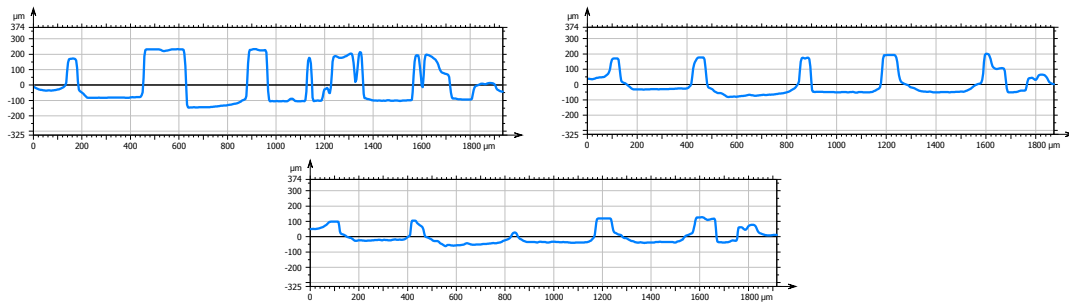
Profils 2D d'une macro-texture sous compressions uniaxiales.
