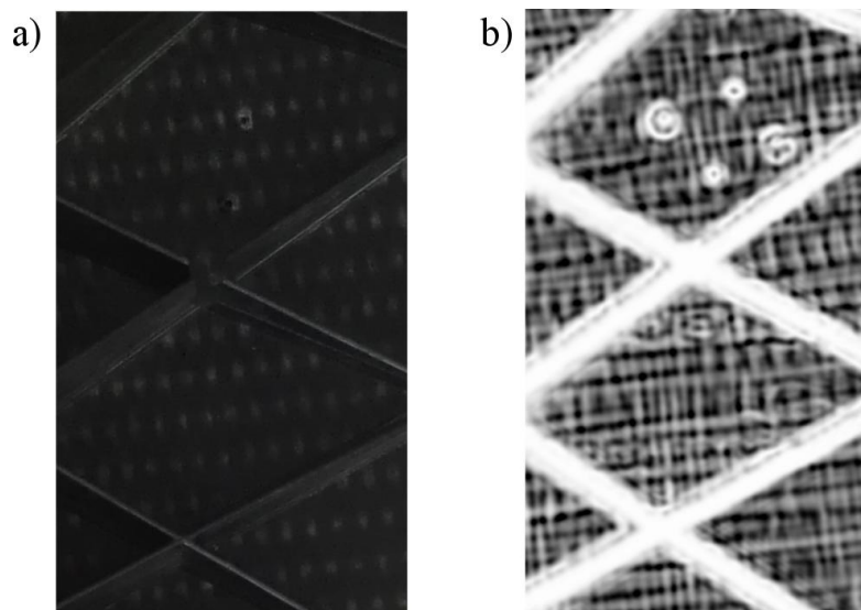
Figure 3 : Pièce composite à renforts tissés issue de l'industrie. a) Photographie de la zone imagée. b) Image de l'intensité THz transmise.
