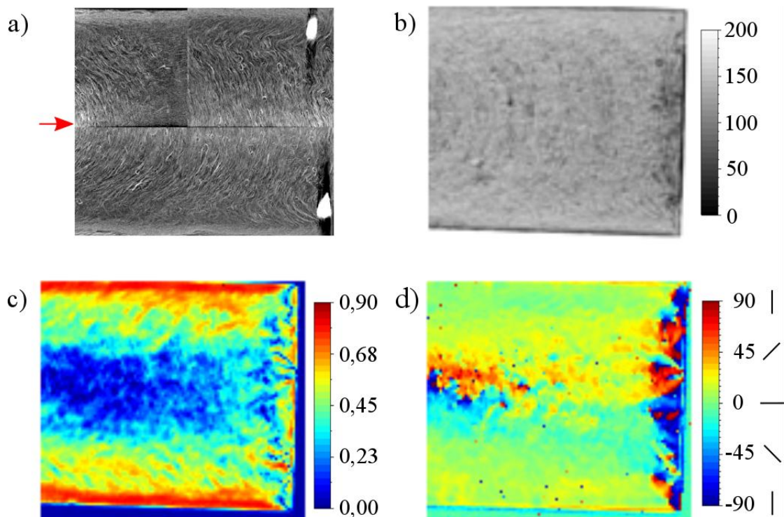
Figure 2 : Résultats plaque de PPGFL 40% sur une zone d'observation de 210mm*190mm : a) Coupe par tomographie par rayons X dans la veine centrale. La flèche rouge représente la position du point d'injection. b) Intensité THz transmise (mV). c) Magnitude de l'anisotropie optique. d) Orientation du grand axe de l'anisotropie optique (degrés).
