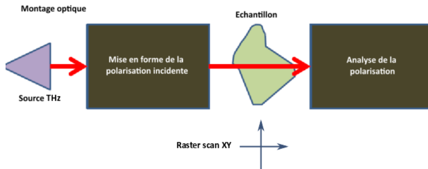
Figure 1 : Schéma du principe de mesure par imagerie polarimétrique THz en transmission.
