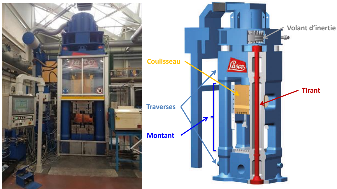
Figure 1 : Photo et schéma de la presse à vis Lasco SPR 400 de la plateforme Vulcain
